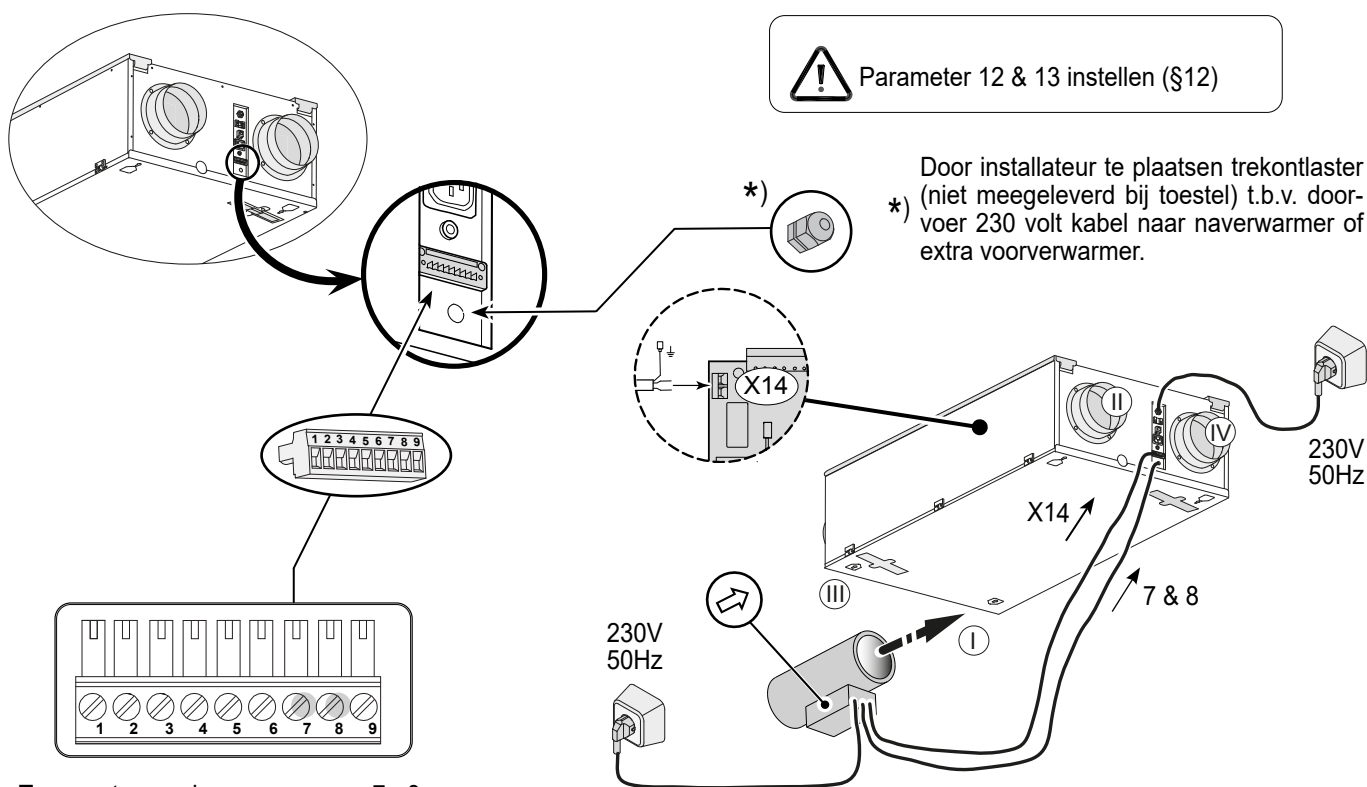
Temperatuurvoeler naverwarmer 7 - 8.
